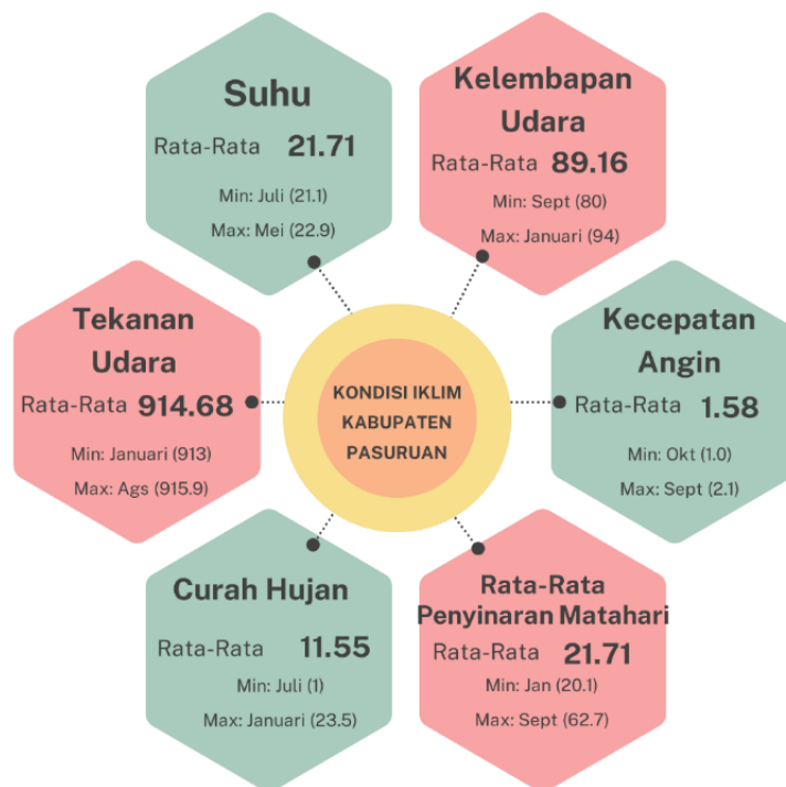
Gambar 2.3 Iklim Kabupaten Pasuruan
