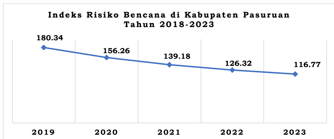
Gambar 2.9 Indeks Risiko Bencana di Kabupaten Pasuruan Sumber : Badan Penanggulangan Bencana Daerah Kabupaten Pasuruan, 2024
