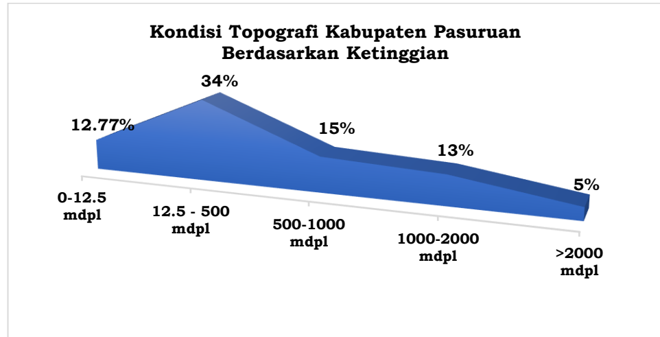
Gambar 2.2 Kondisi Topografi Kabupaten Pasuruan Berdasarkan Ketinggian
