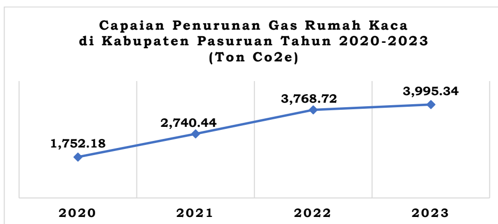
Gambar 2.11 Capaian Penurunan GRK Kabupaten Pasuruan Sumber : BAPPELITBANGDA Kabupaten Pasuruan, 2024 (AKSARA, 21 Mei 2024)
